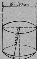
Croquis coté de la masse TARE = 60Kgs ± 0 Kg 200
