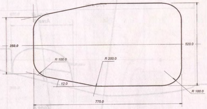
Fig. 2 : Cockpit entry template / Gabarit d'entrée de l'habitacle
