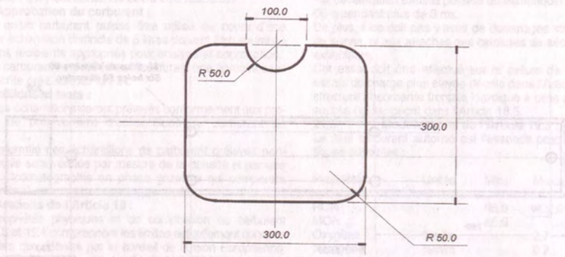
Fig. 3 : Cockpit cross section template / Gabarit de section de l'habitacle
