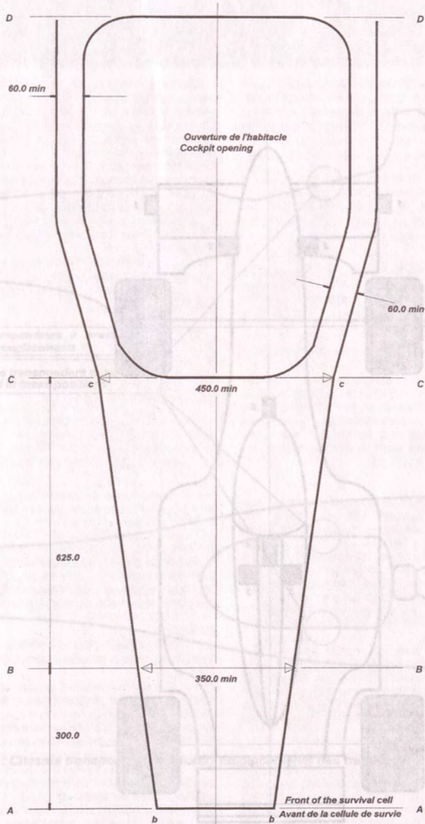
Fig. 5 : Survival cell dimensions / Dimensions de la cellule de survie
