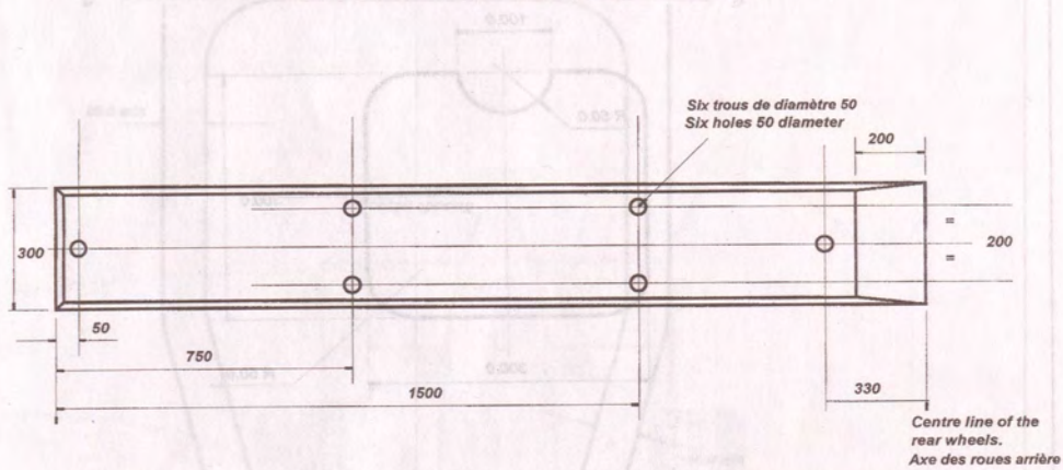
Fig.1 : Skid block dimensions / Dimensions du patin
