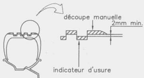
Dessin No 290-2
