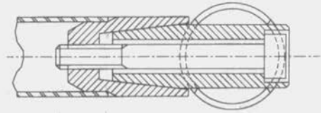
Dessin No 253-29
