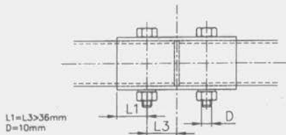
Dessin No 253-32
