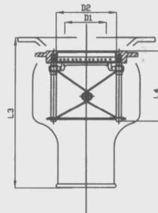
Prise femelle
