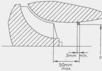
Dessin No 285-1
