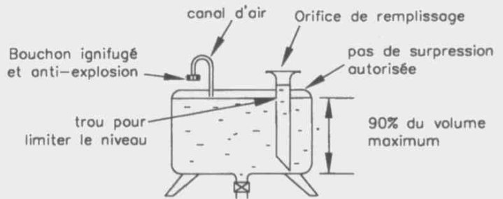
Dessin No 252-3
