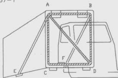
Dessin No 287-3
