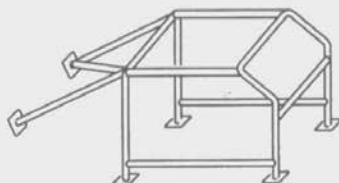
Dessin No 283-6
