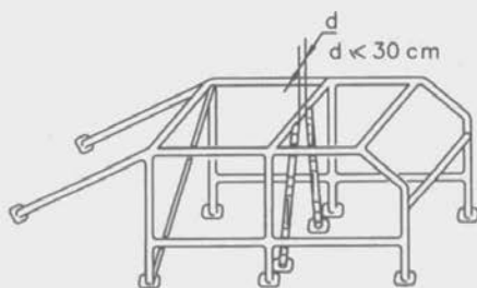
Dessin No 283-5
