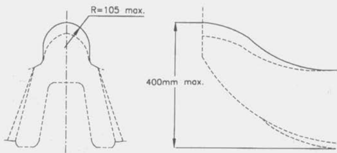
Dessin No 262-7
