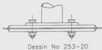
Dessin No 253-20
