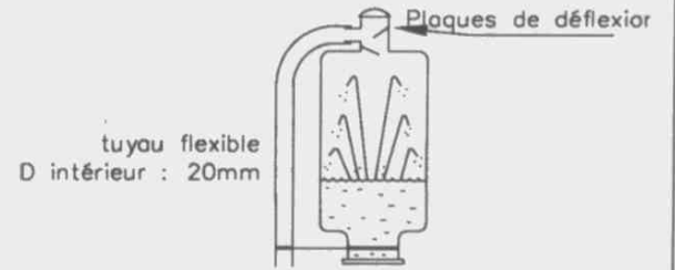
Dessin No 252-1
