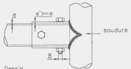
Dessin No 253-34
