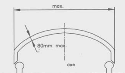
Dessin No 258-1
