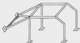
Dessin No 253-14
